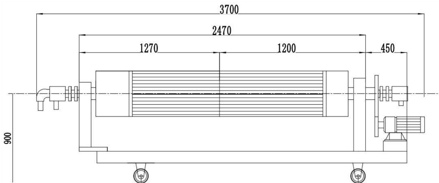
正视图 FRONT VIEW
